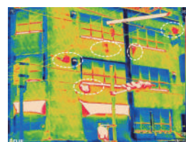
外壁劣化の赤外線画像
