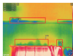
雨漏り診断の赤外線画像
